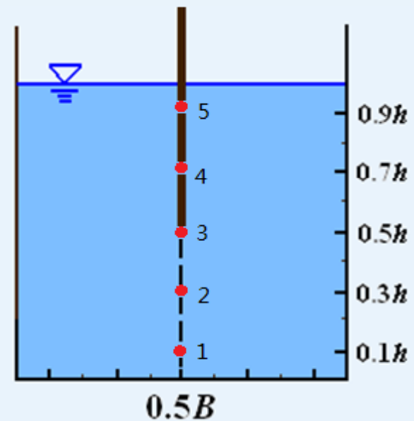
垂直面上流速
