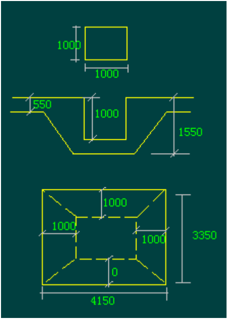
图 2.21-2: 软件设置集水井
