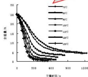
图 1 初含湿量 25% 的干燥曲线 (小五宋体, 居中)
