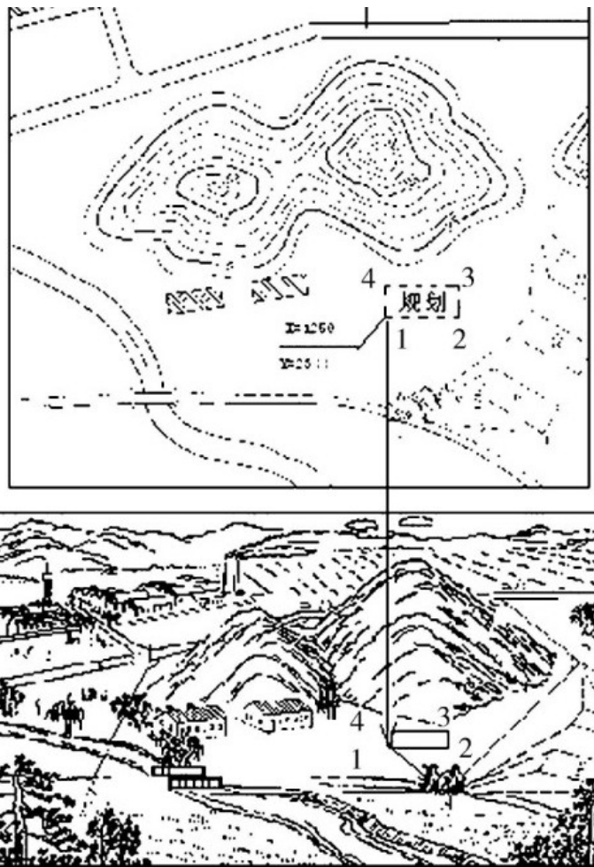
测设示意图
