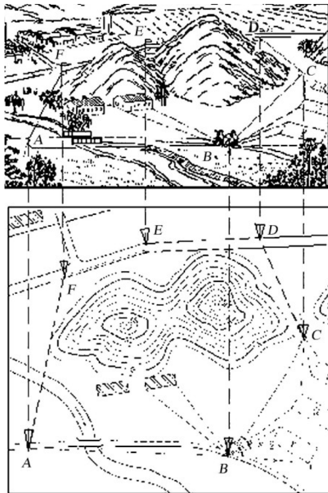
测定示意图
