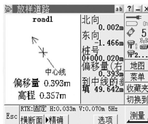
图10-21 实时线路建立
