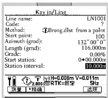
图10-20 放样线路建立
