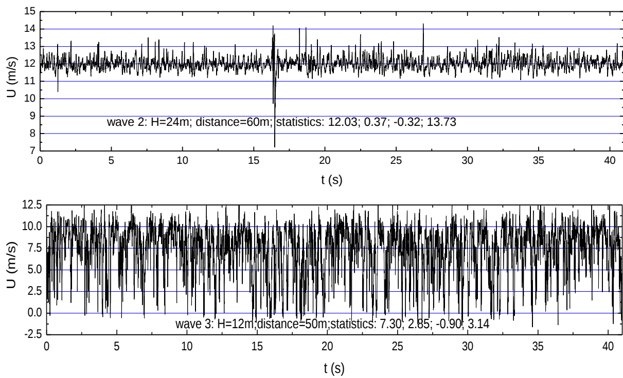
图 2-7 典型脉动风速时程
