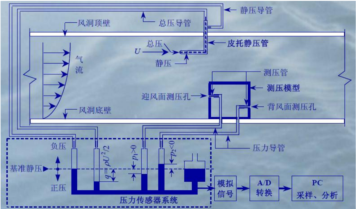
图 2-18 风洞测压试验流程示意图
