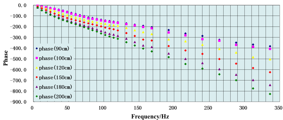
图 2-27 不同条件下信号相位差
