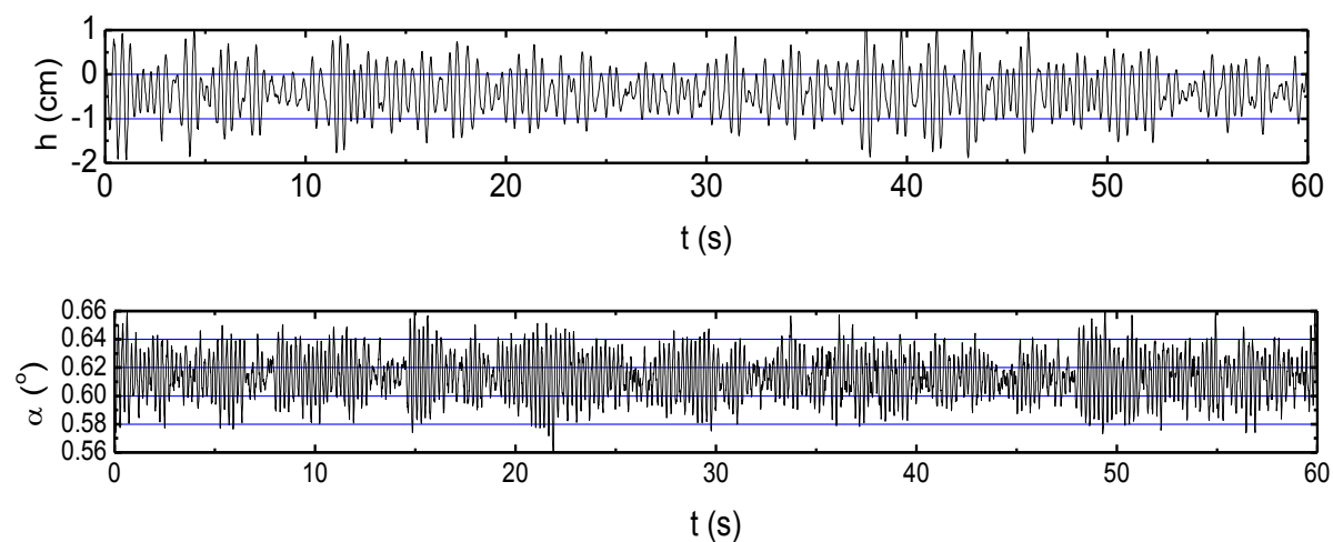
图 2-11 模型振动位移时程
