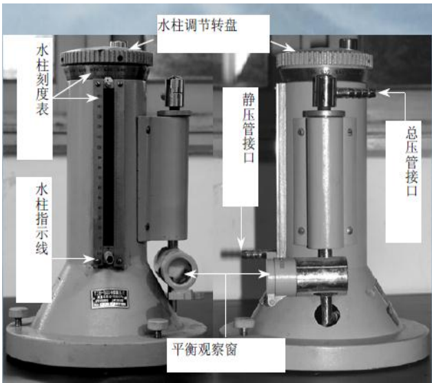
图 2-2 微压计
