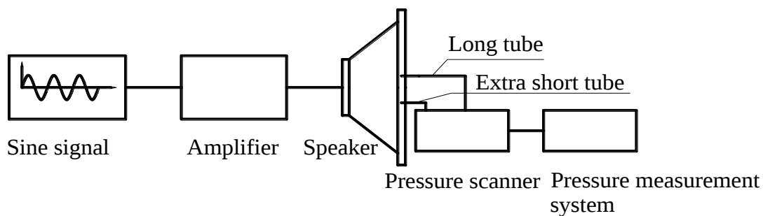
图 2-24 压强标定系统示意图
